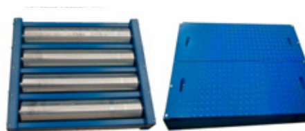
Fig. 1.- Kit rodillos libres para vehículos industriales de doble carro.
